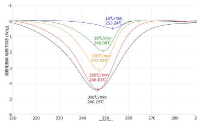
図 ポリエチレンテレフタレート(PET)のDSC測定結果 試料量:0.5mg、加熱温度:10℃/min,50℃/min, 100℃/min,200℃/min,300℃/min
