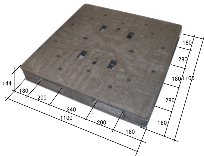
寸法図
